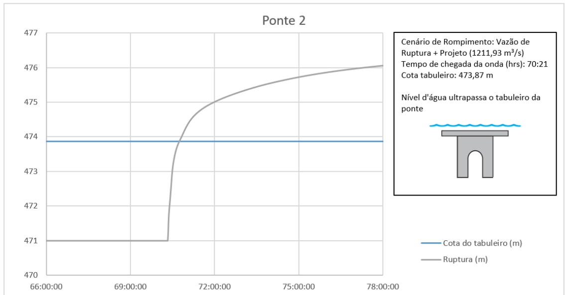
Figura 17 – Cotagrama da Ponte 2
