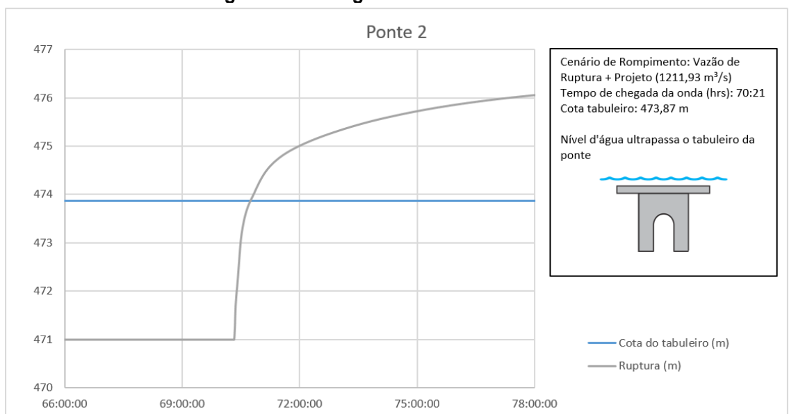
Figura 36 – Cotograma da Ponte 2
