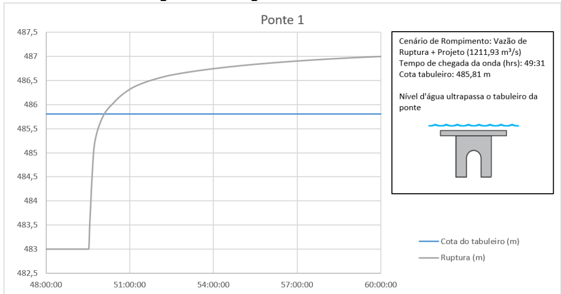
Figura 25 – Cotograma da Ponte 1
