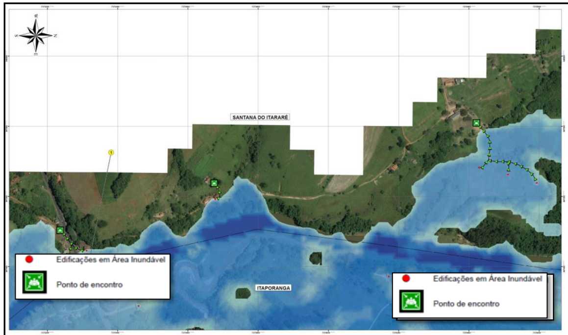
Figura 24 – Identificação da ZSS 24 em Santana do Itararé – PR
