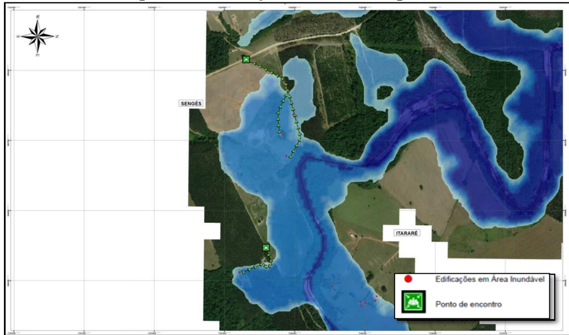
Figura 14 – Identificação da ZSS 08 em Sengés – PR
