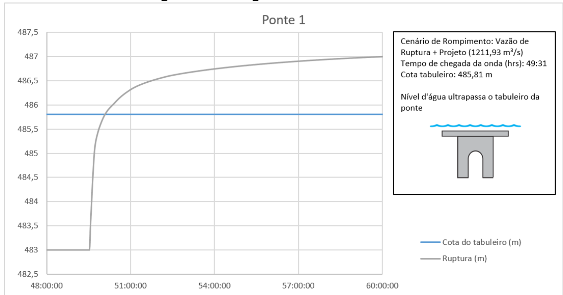
Figura 18 – Cotograma da Ponte 1
